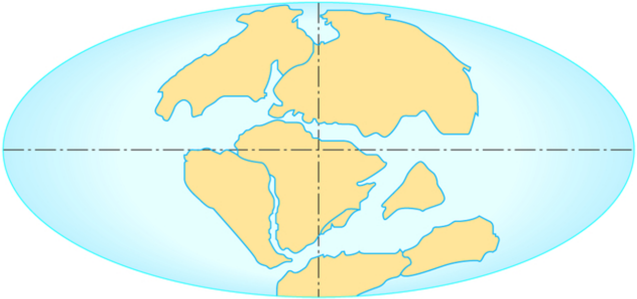
La Terre, il y a 130 millions d'années
